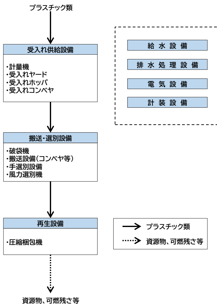
図 3.28 プラスチック類資源化施設の基本処理フロー（案）
